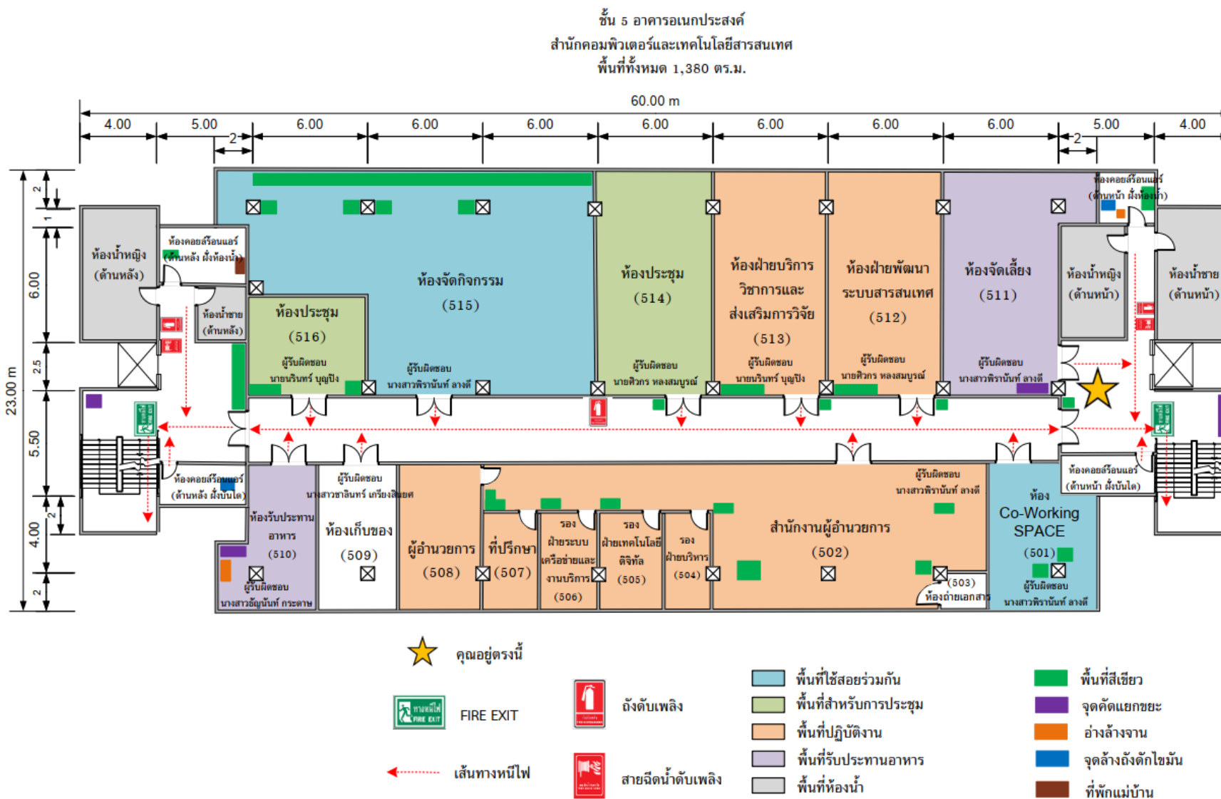
แผนผังทางหนีไฟชั้น 5 อาคารอเนกประสงค์
